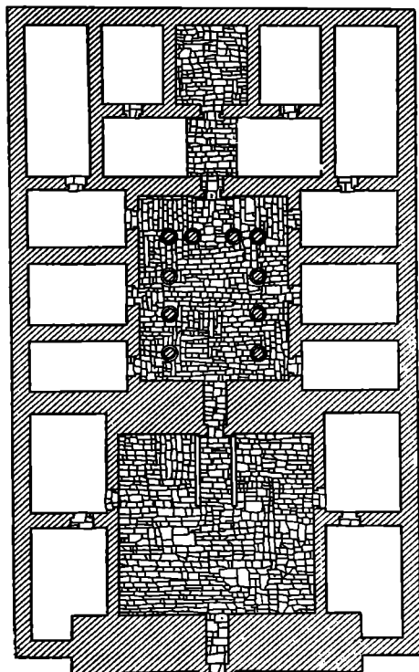
Рис. 7. Северный анонимный храм. План (A. Varille — С. Robichon, табл. XIII)
