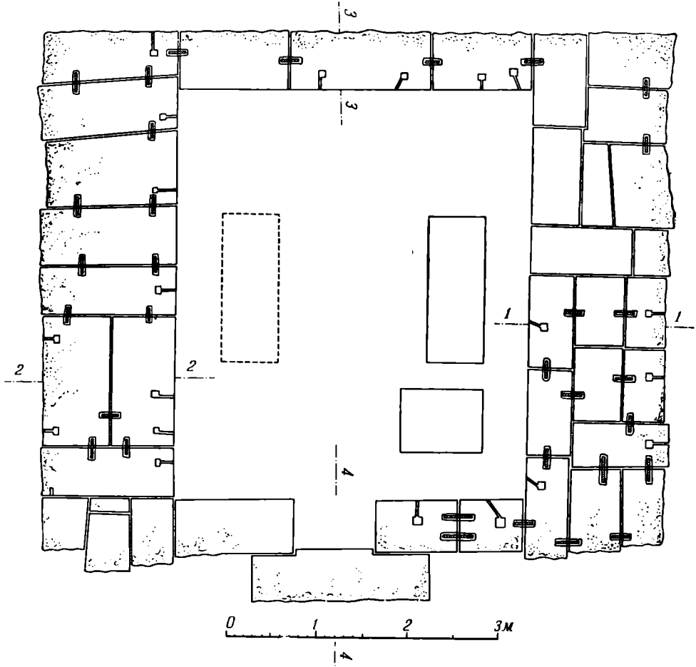
Рис. 2. Горизонтальный разрез склепа
