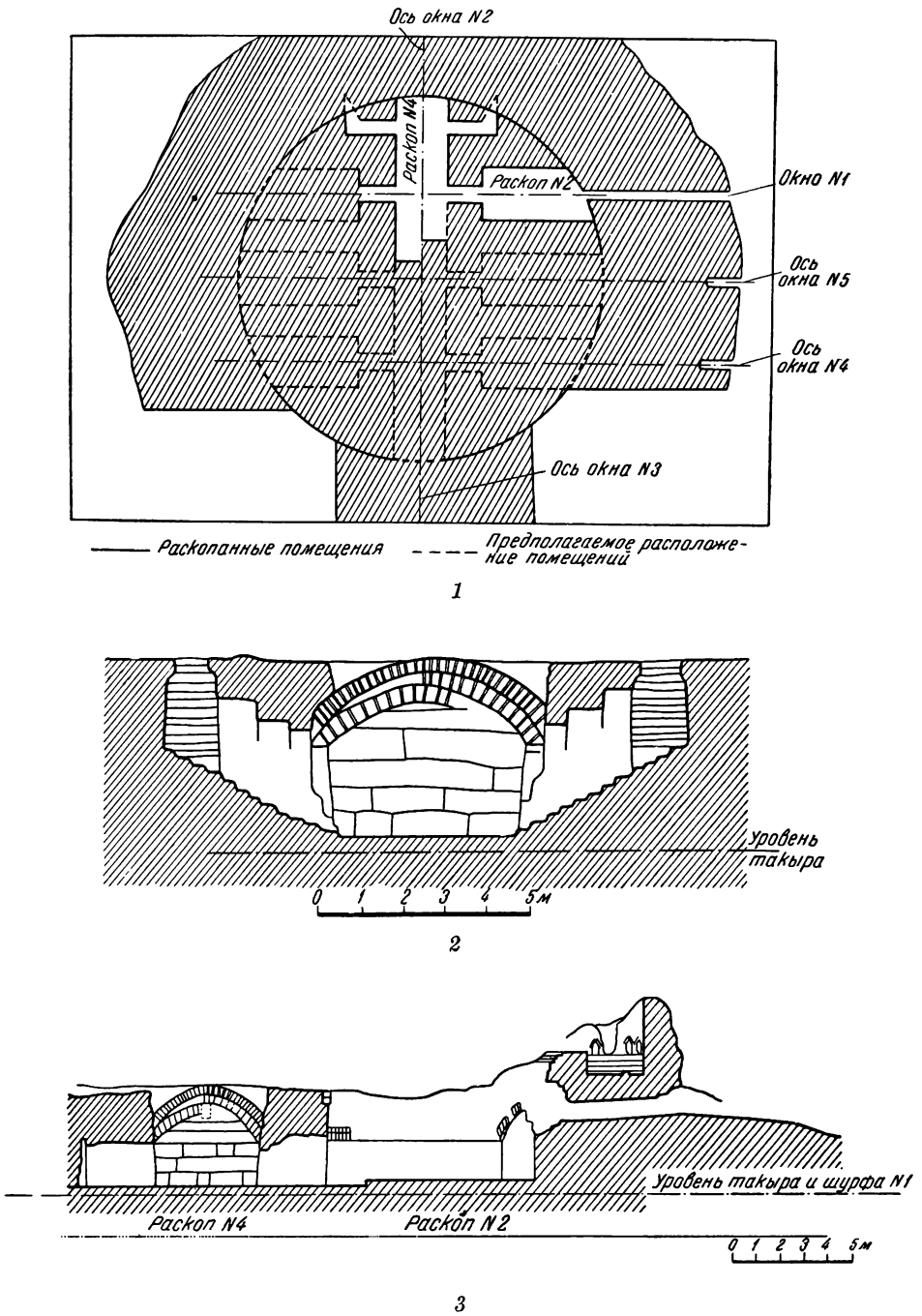
Рис. 5. Схема размещения нижних помещений Центральной площадки (1) и разрезы через помещения №№ 2 и 4 (2, 3' (обмеры арх. М. С. Лапирова-Скобло)
