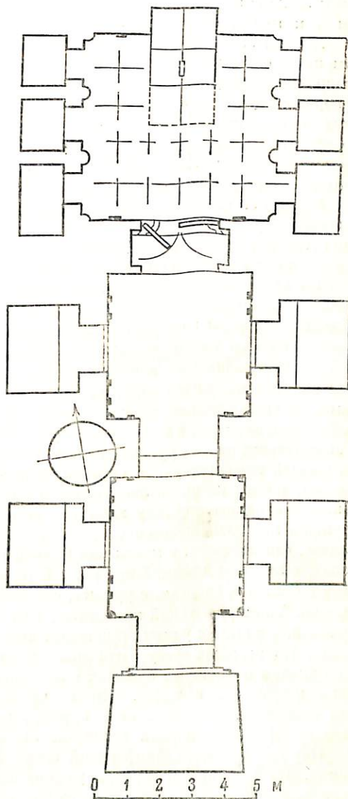
Рис. 4. План кургана императора Лишэна
