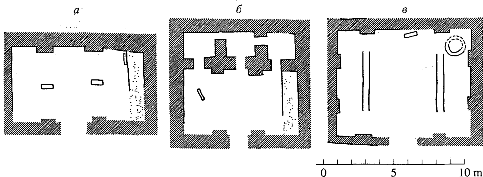
Рис. 1 а–в. а – Чейёню Тепеси. План «Здания с плитами»; б – Чейёню Тепеси. План «Дома черепов»; в – Чейёню Тепеси. План «Здания с мозаичным полом» (по: Hauptmann H. Ein Kultgebäude in Nevalı Cori // Between the Rivers and Over the Mountains. Roma, 1993. P. 67. Add. 28)
