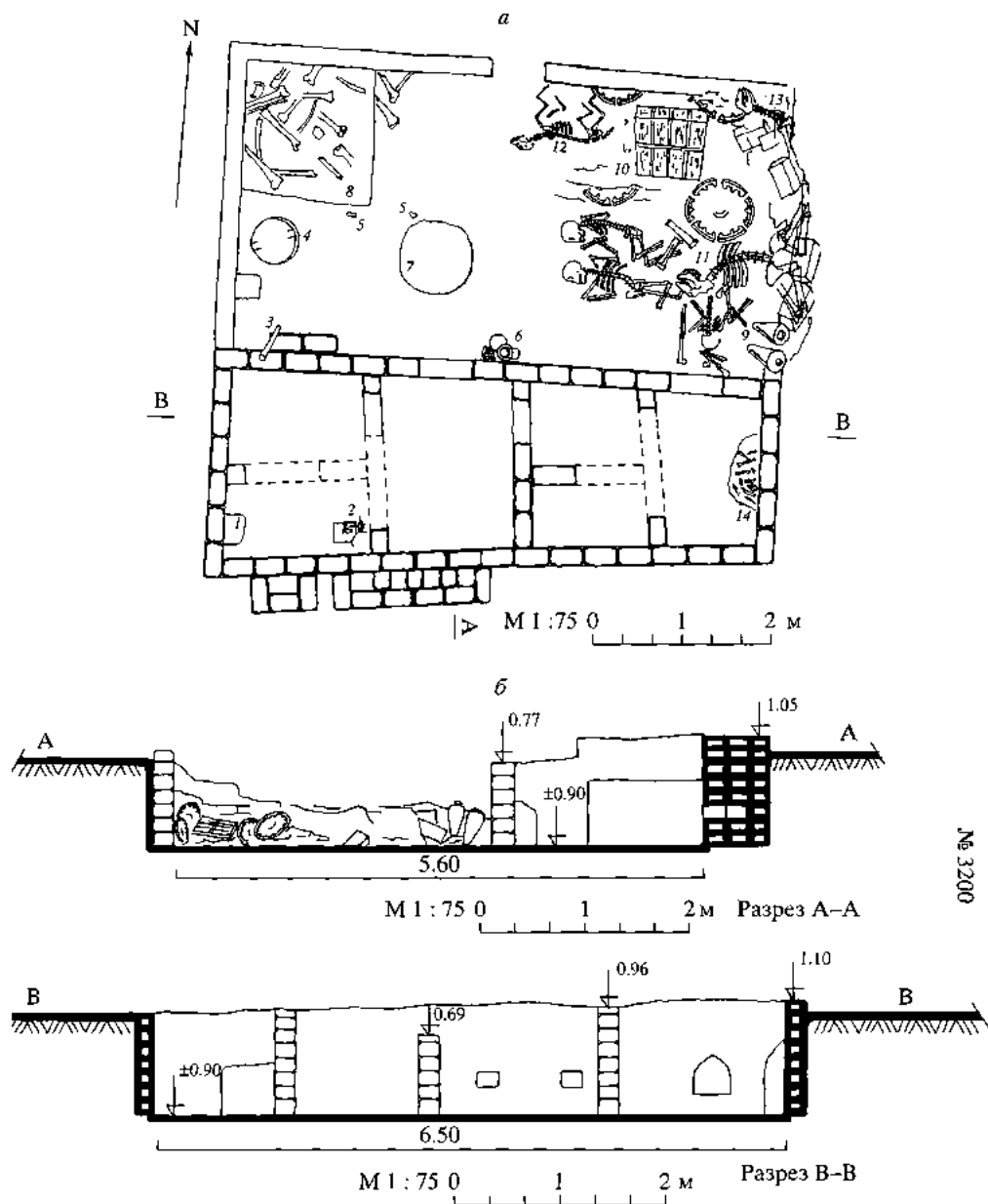
Рис. 2. Гробница № 3200. а – План. 1 – скопление ценных погребальных привошений; 2 – два фрагмента мозаики с «ковровым» орнаментом, серебряные косметический флакон, косметическая лопаточка, булавка с навершием в виде лежащего теленочка, железная булавка с навершием в виде золотой восьмиконечной звезды, полумесяца, а также стоящего архара из золота и лежащего льва из бирюзы; 3 – каменный посох длиной 2.0 м с концом в виде лошадиного копыта; 4 – каменный диск из мраморизованного известняка; 5 – бронзовые предметы неопределенного назначения; 6 – два бронзовых «светильника» и керамическая ваза на полной ножке с орнаментом; 7 – лянто из краснообожженного песка; 8 – скопление костей взрослого верблюда; 9 – два крупных керамических сосуда с узким дном; 10 – четырехколесная повозка; 11 – скелет лежащего взрослого верблюда в полном анатомическом порядке; 12 – полный скелет собаки в полном анатомическом порядке; 13 – сильно разрушенный скелет молодой лошади; 14 – беспорядочное скопление костных останков четырех человек; б – разрезы
