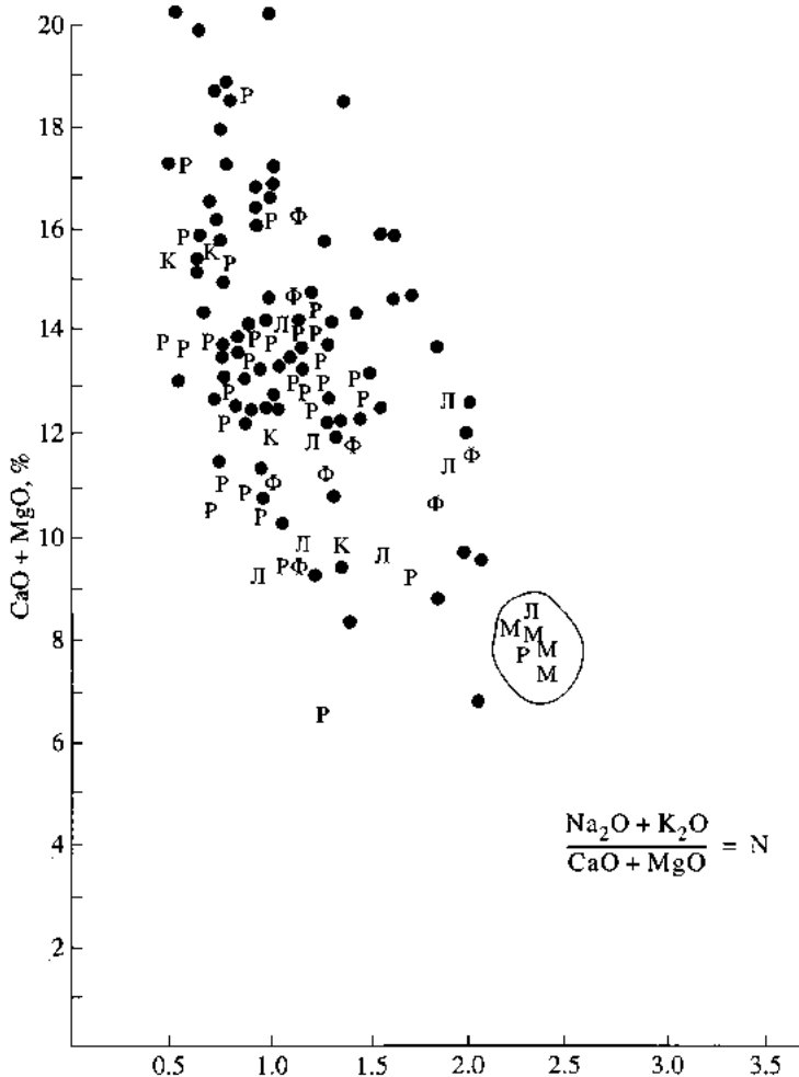
Рис. 10. Количественно-качественная характеристика стекол V–I вв. до н.э., сваренных по античному рецепту. К – «кулоны», Л – лятиксы-скарабеиды, Р – рубчатые бусы, Ф – фиалы, • – массовый материал. М – «мокрый» анализ
